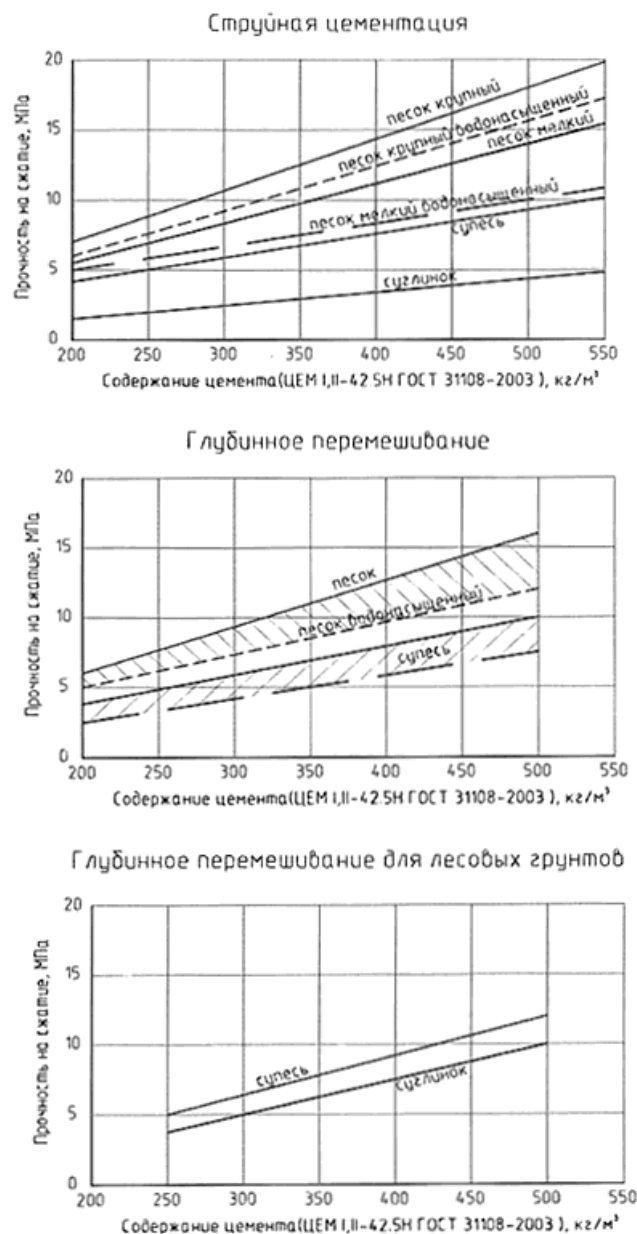
Рисунок Ф.3 - Зависимость прочности грунтоцемента от содержания цемента в 1 м³ ГЦЭ
