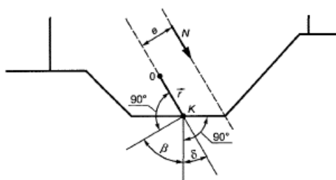
Рисунок Л.1 - Схема к определению нормальных и касательных контактных напряжений при ломаной
