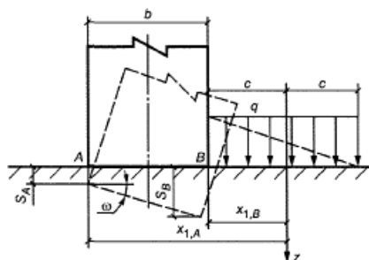
Рисунок 2 - Схема к определению крена сооружения от пригрузки
