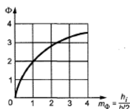
Рисунок С.2 - График для определения коэффициента \Phi
