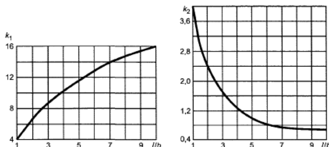
Рисунок 1 - Графики для определения коэффициентов k_1 и k_2
